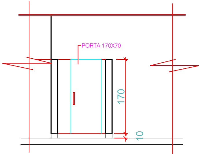
DETALHE 1- PAREDE E PORTA BANHEIRO
